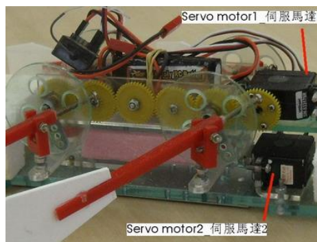
伺服马达 2：作左右摆动
