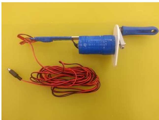
24V 350 rpm 手搖發電裝置
