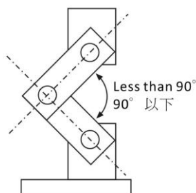
少于 90 度單轉軸膝關節設計
