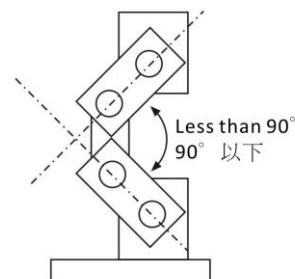
少于 90 度雙轉軸膝關節設計
